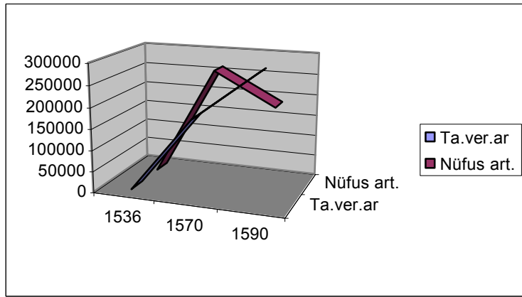
Şekil 2: Ürün-Nüfus Grafiği
